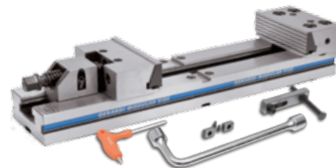
Art.150 prismatica sovrapponibile
